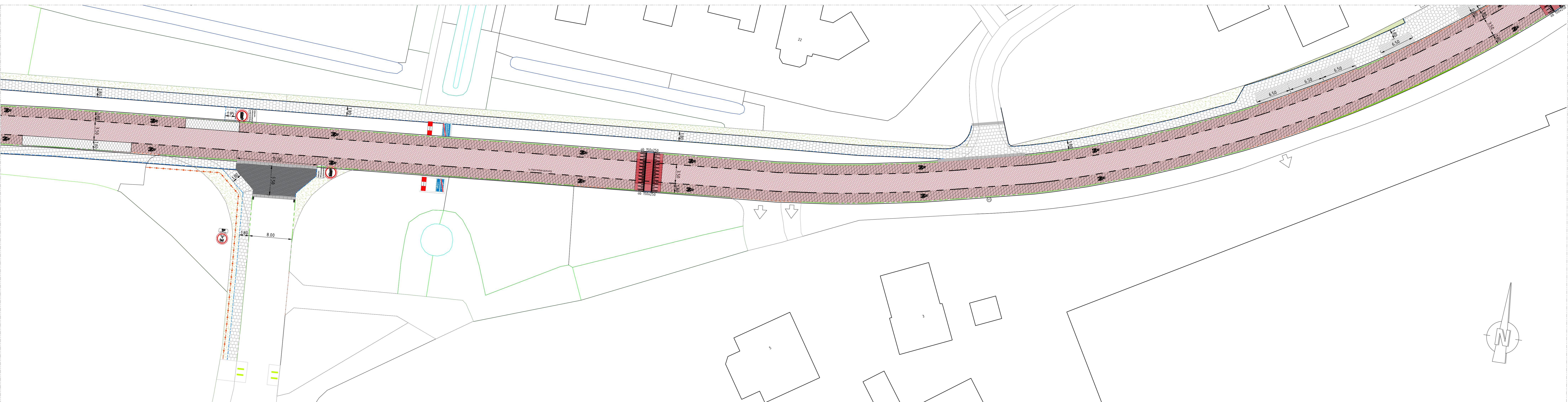
Lengelseweg wegvak 1b schaal 1:250
